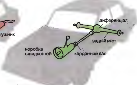
Привідний механізм
